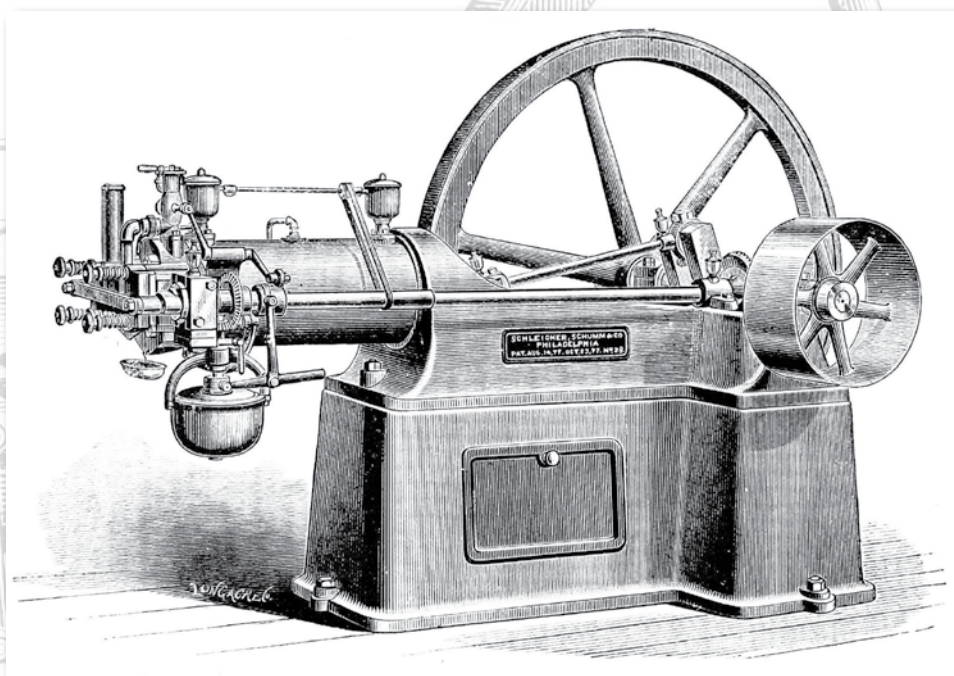
Αμερικανική μηχανή εσωτερικής καύσεως Όττο (1880).
